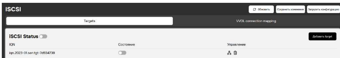
Рисунок 70 – Протокол iSCSI
