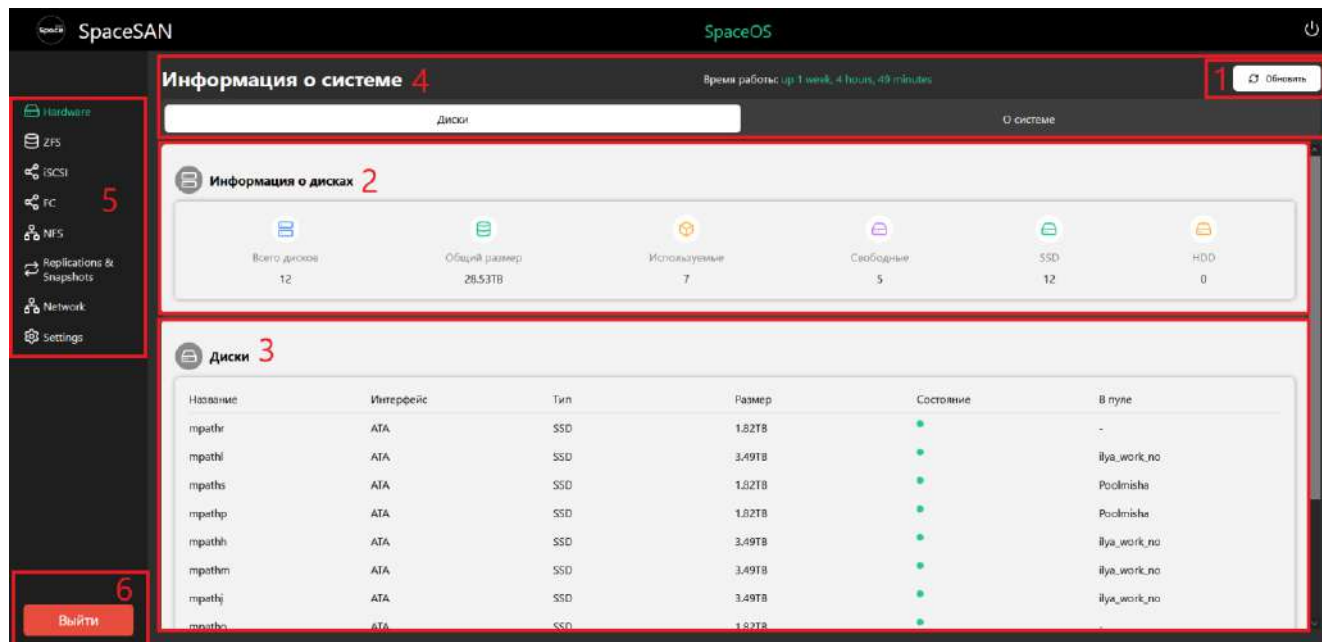
Рисунок 23 – Главный экран
