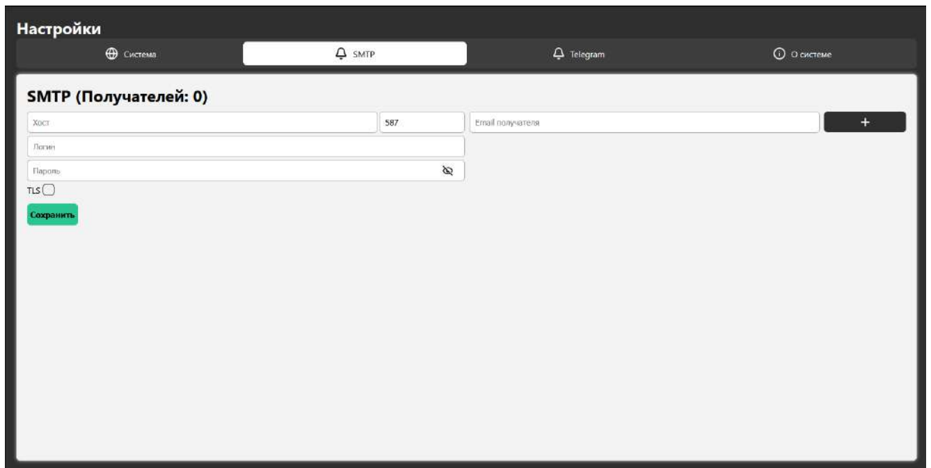
Рисунок 100 – Вкладка «SMTP»
