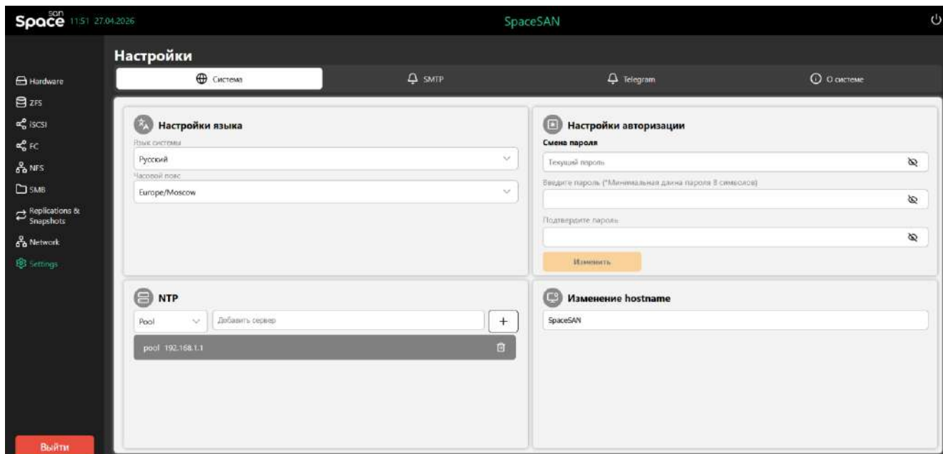
Рисунок 97 – Раздел «Настройки»
