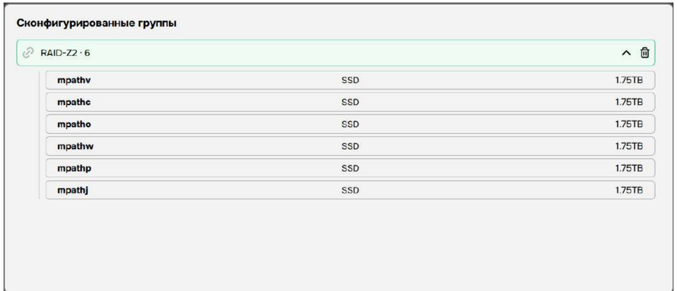
Рисунок 33 – Выбранные диски
