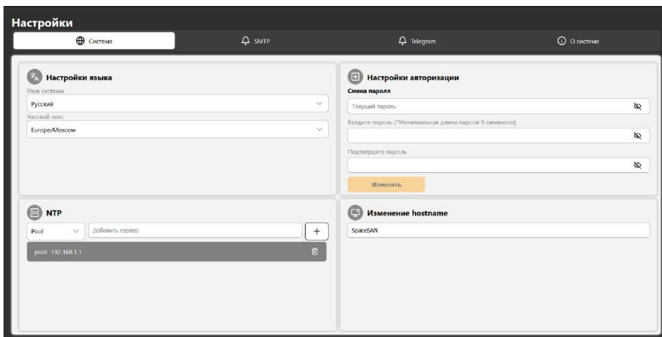
Рисунок 98 – Вкладка «Система»
