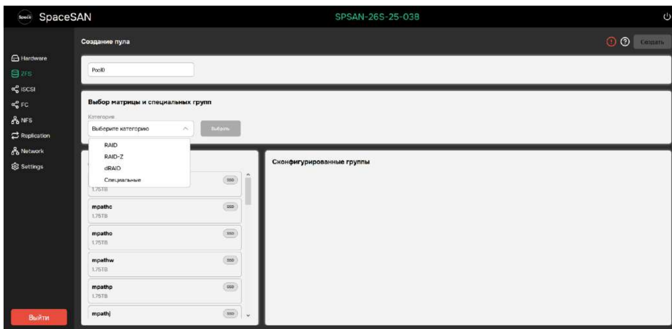
Рисунок 29 – Выбор категории
