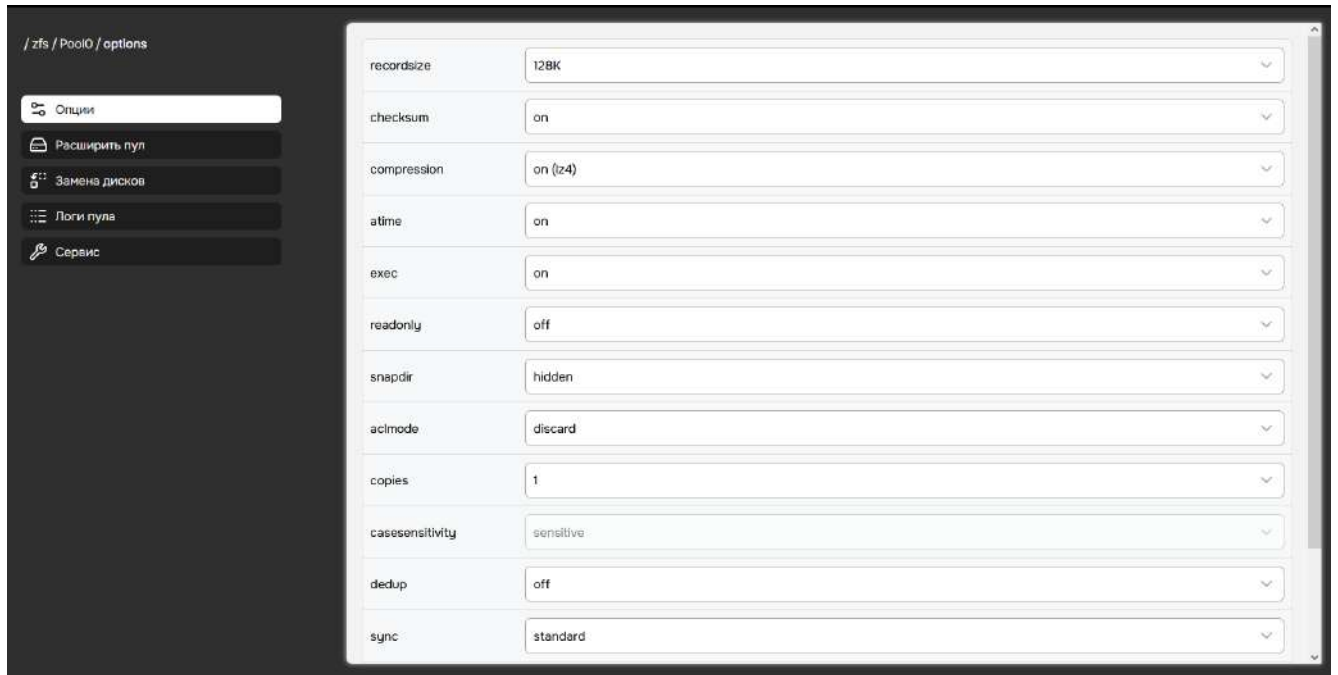
Рисунок 38 – Параметры пула
