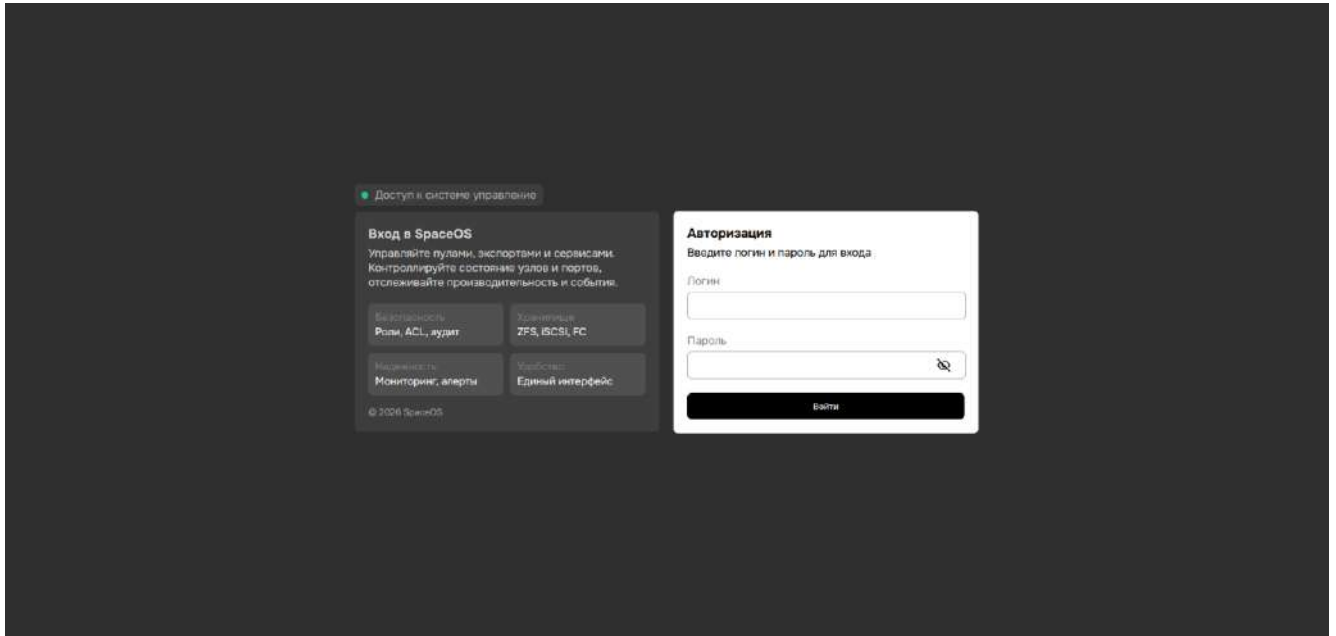
Рисунок 21 – Авторизация
