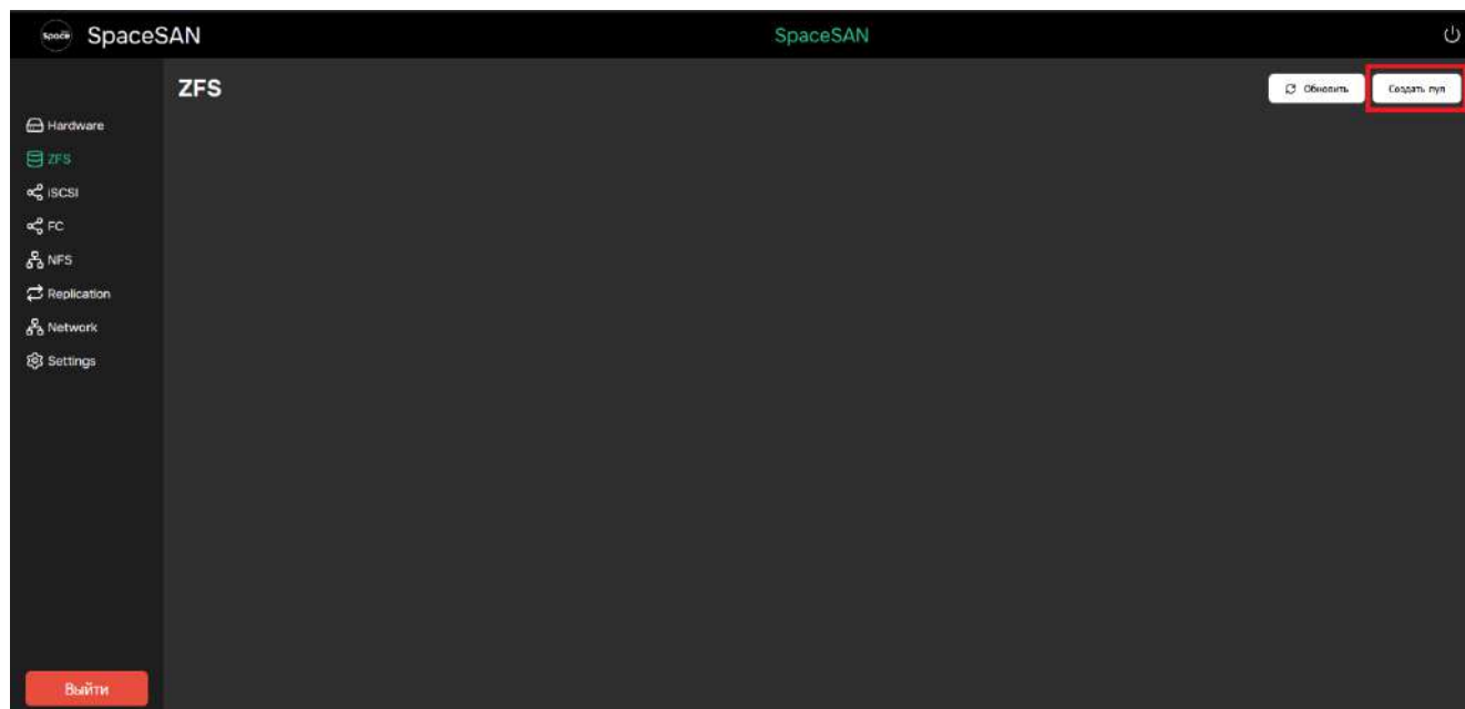
Рисунок 27 – Вкладка ZFS
