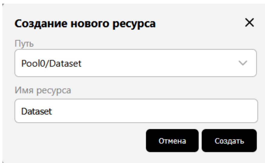
Рисунок 78 – Создание SMB-ресурса
