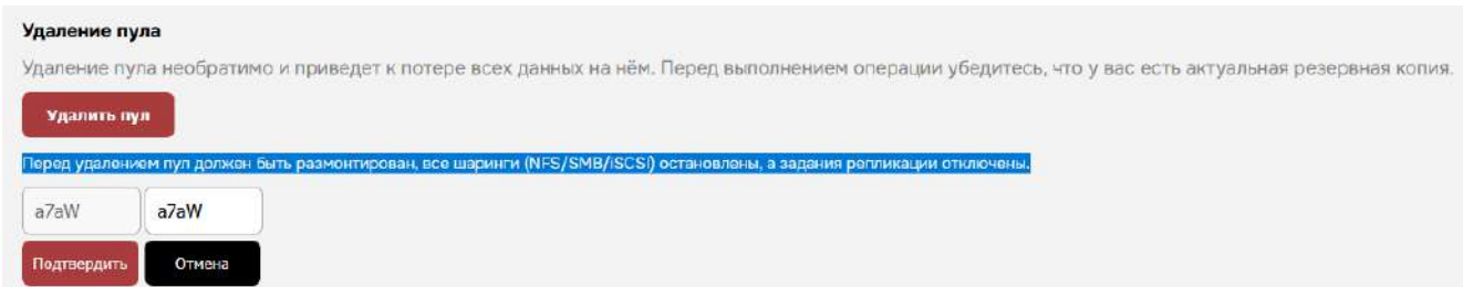
Рисунок 46 – Удаление пула
