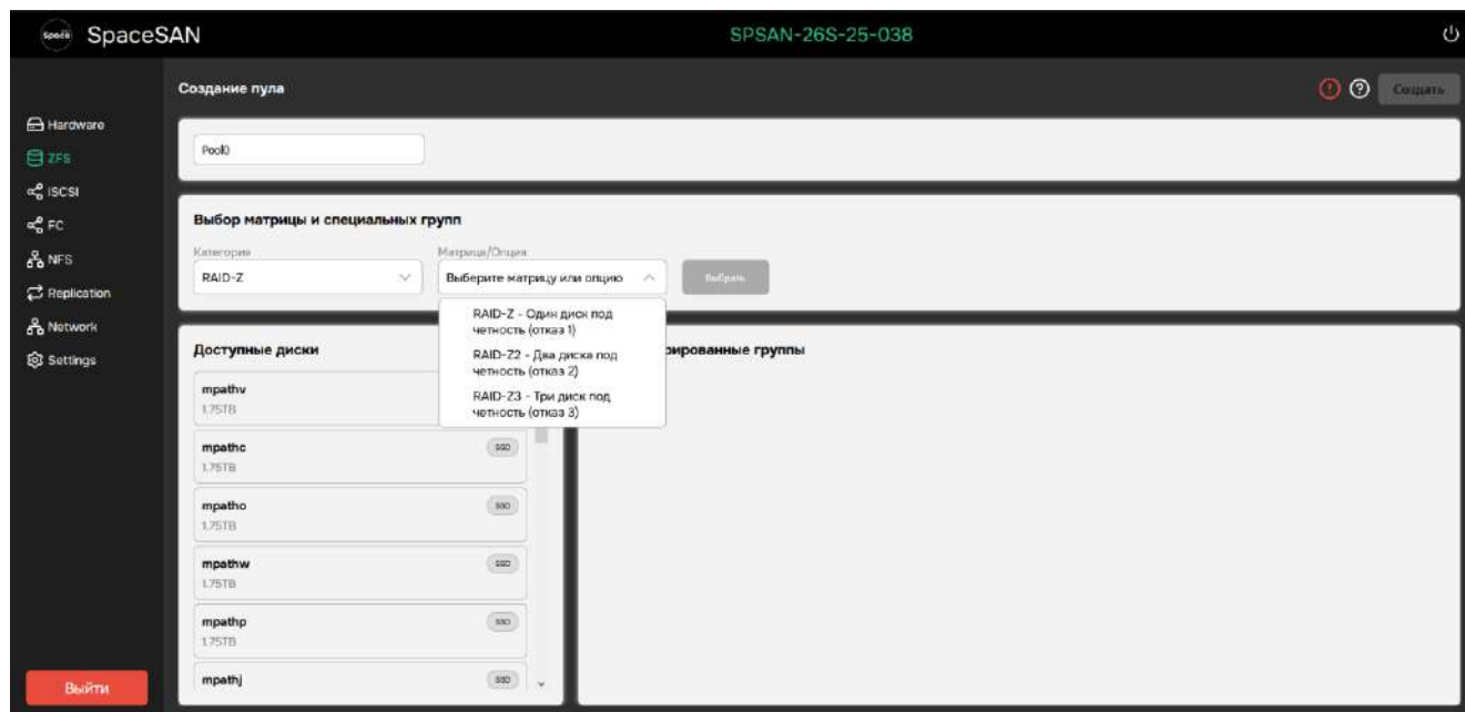
Рисунок 30 – Выбор матрицы/опции
