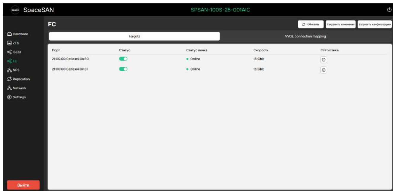
Рисунок 62 – Fibre Channel
