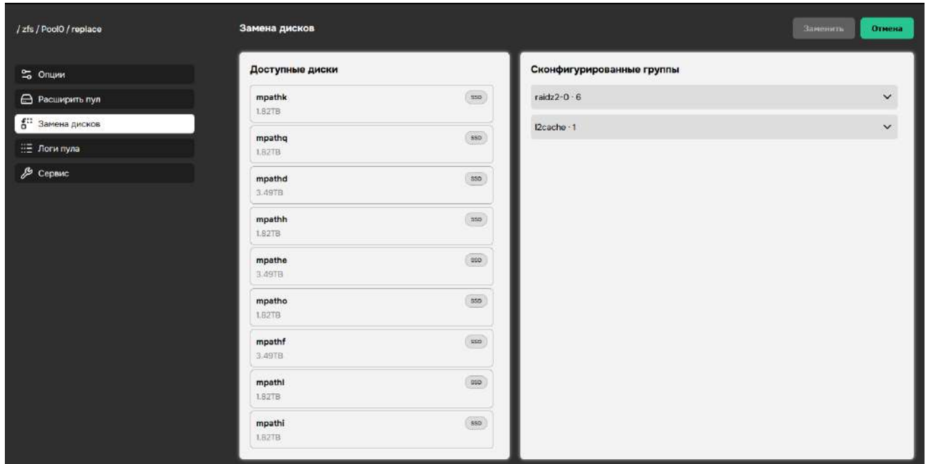
Рисунок 40 – Замена дисков
