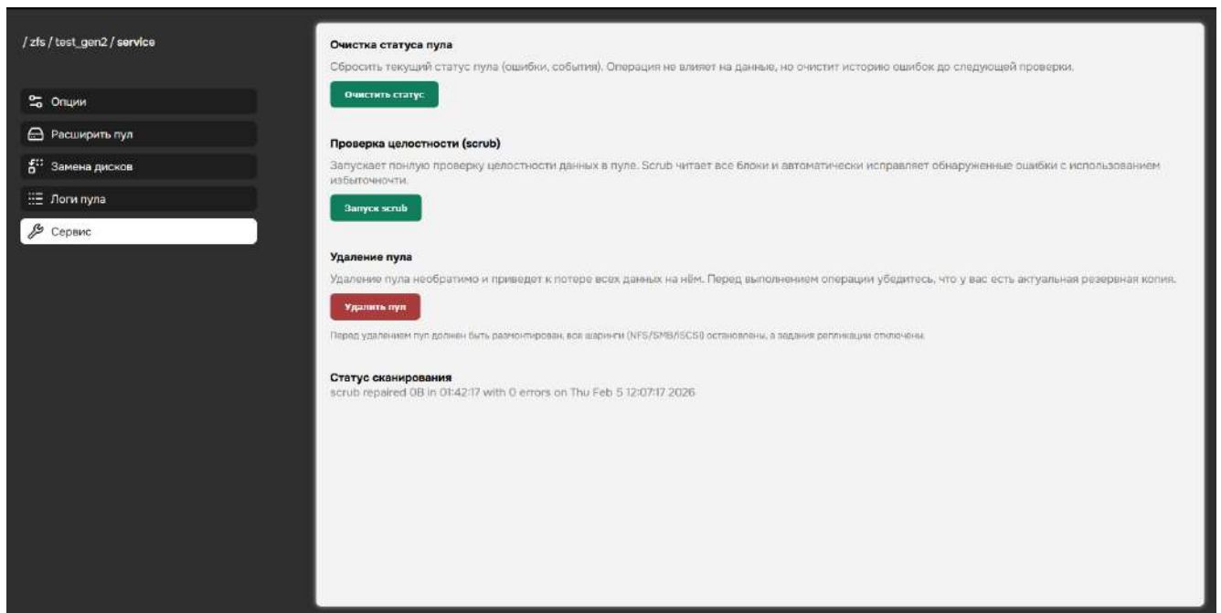
Рисунок 43 – Раздел «сервис»
