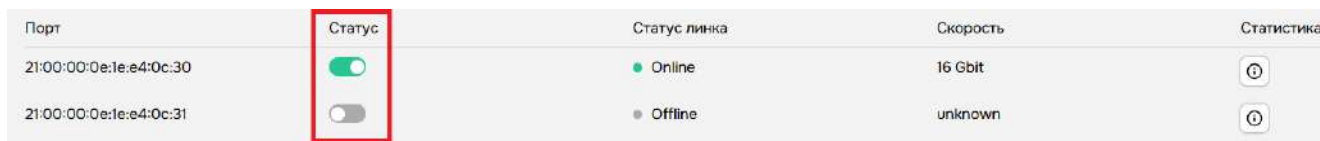
Рисунок 64 – Активация порта
