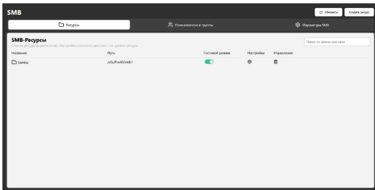
Рисунок 77 – Раздел SMB
