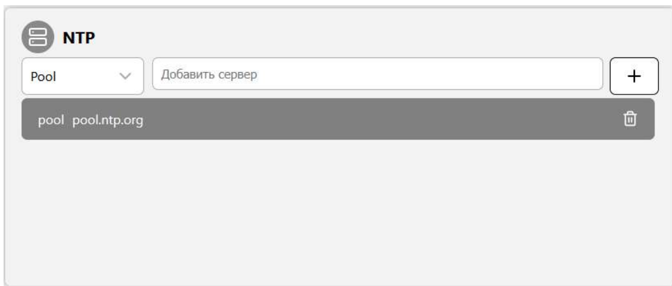
Рисунок 99 – Настройка «NTP»
