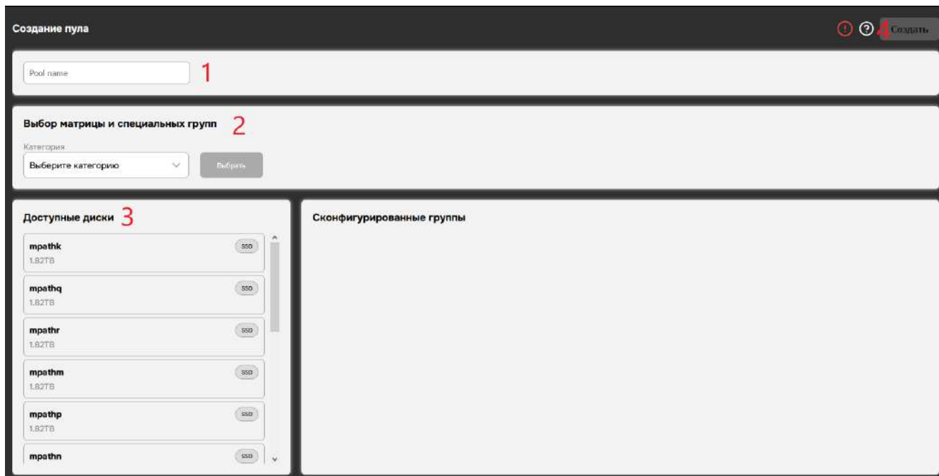
Рисунок 28 – Создание пула
