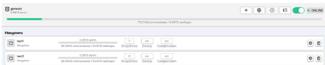
Рисунок 54 – Набор данных
