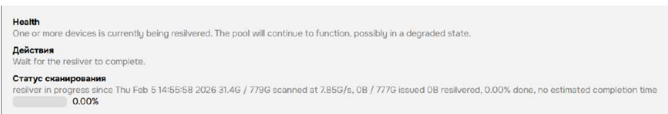
Рисунок 47 – Статус сканирования
