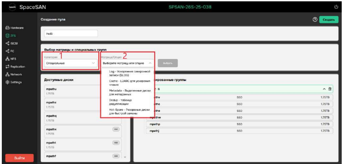
Рисунок 34 – Расширенные опции
