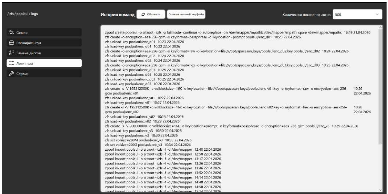
Рисунок 42 – Логи пула
